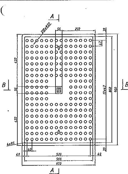
Капак за КАБЕЛНИ ШАХТИ поглед отгоре
